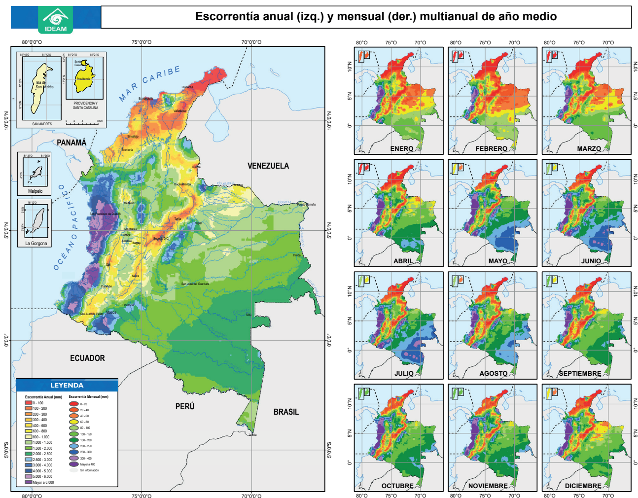
Figura 6. Escorrentía anual (izq.) y mensual (der.) multianual de año medio.
