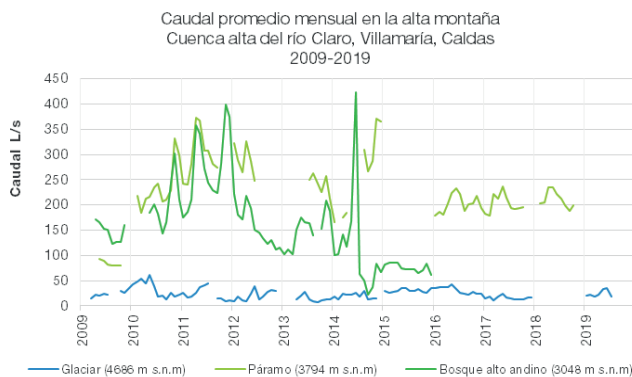
Figura 21. Caudal promedio en los ecosistemas de alta montaña. Casos cuenca Río Claro (izq.), río Cardenillo, Güicán de la Sierra, Boyacá (der.). El caudal de cada ecosistema incluye el (los) del ecosistema inmediatamente superior.
