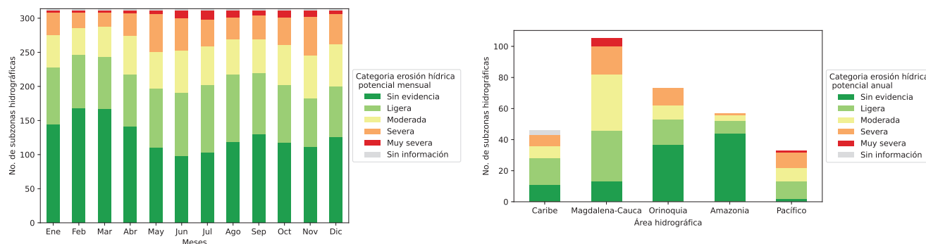
Figura 29. Variabilidad anual de la erosión hídrica potencial (izq.) y número de subzonas según categoría de erosión hídrica potencial por área hidrográfica (der.).
