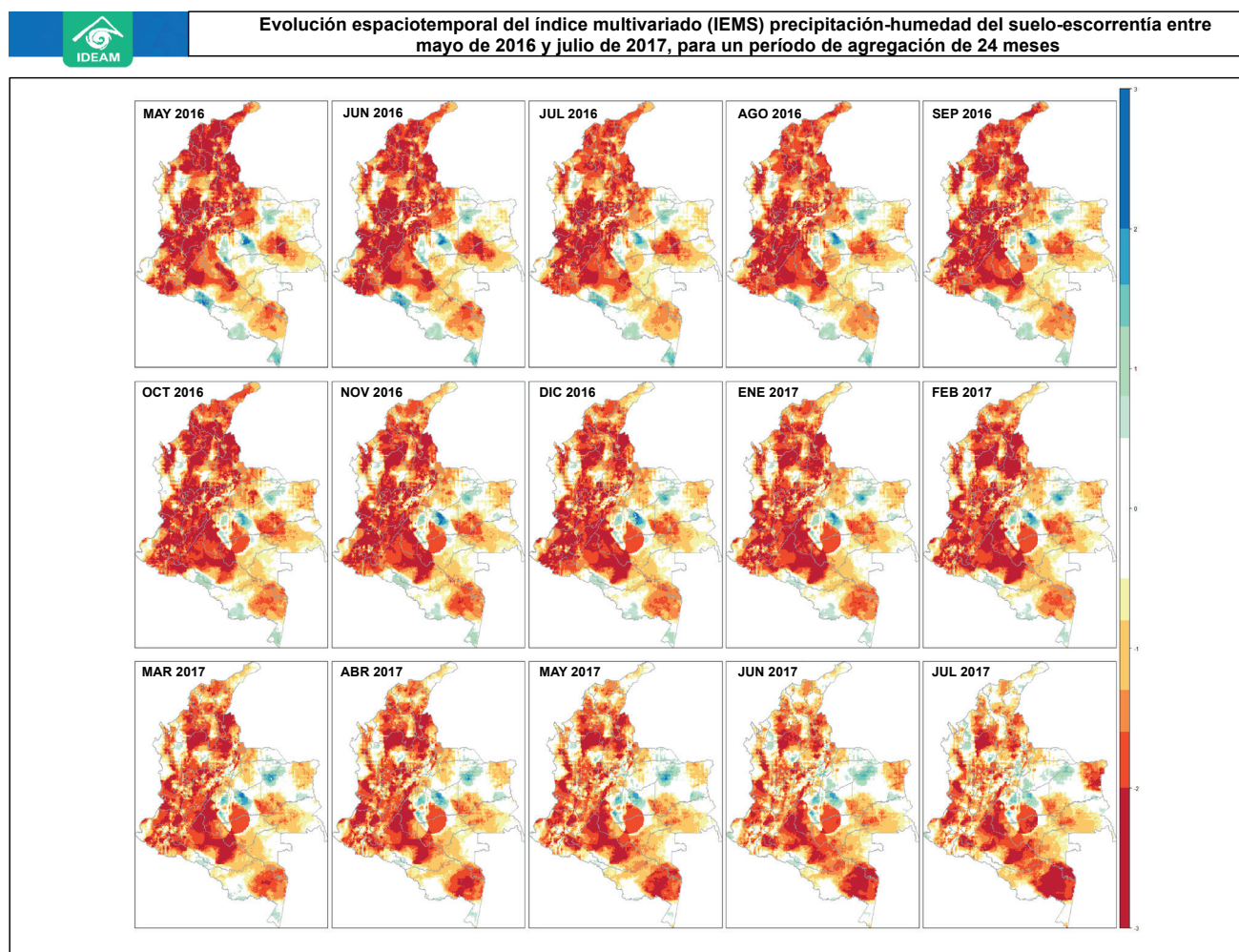
Figura 12. Evolución espaciotemporal del índice multivariado (IEMS) precipitación-humedad del suelo-escurrentía entre mayo de 2016 y julio de 2017, para un periodo de agregación de 24 meses.
