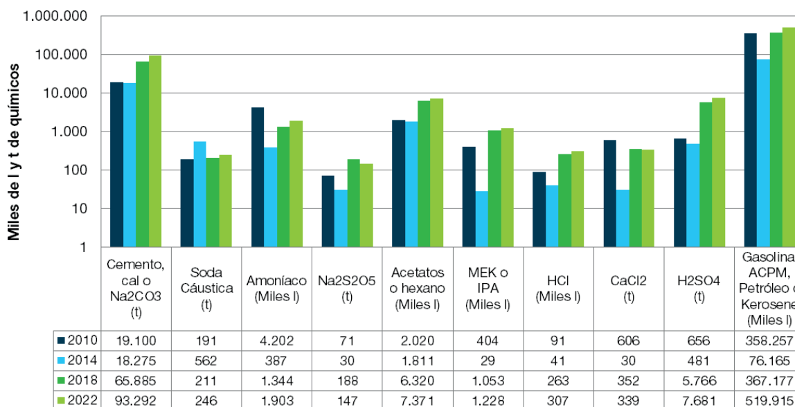
Figura 56. Comparación de sustancias químicas empleadas en la transformación de la coca en Colombia.
