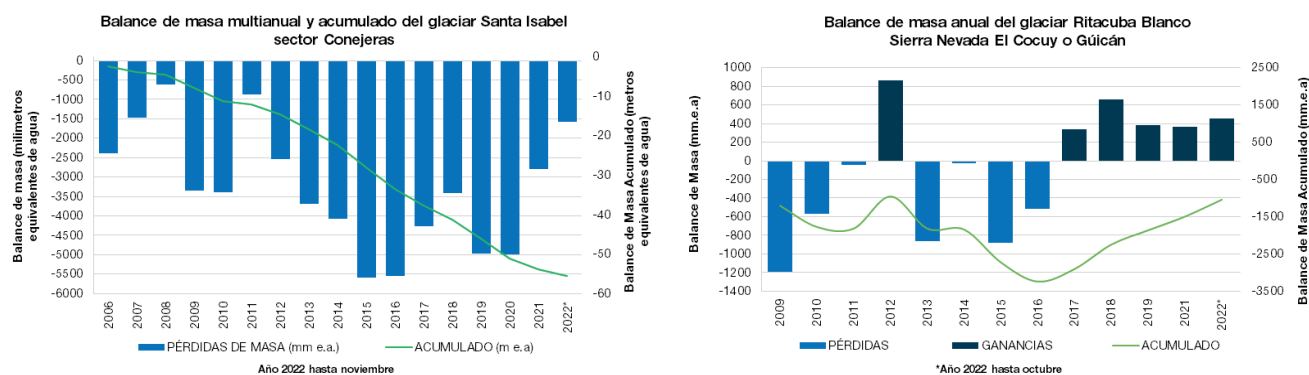
Figura 19. Balances de masa multianual del glaciar Santa Isabel, sector Conejeras (izq.) y de la Sierra Nevada El Cocuy o Güicán, sector Ritacuba Blanco (der.).
