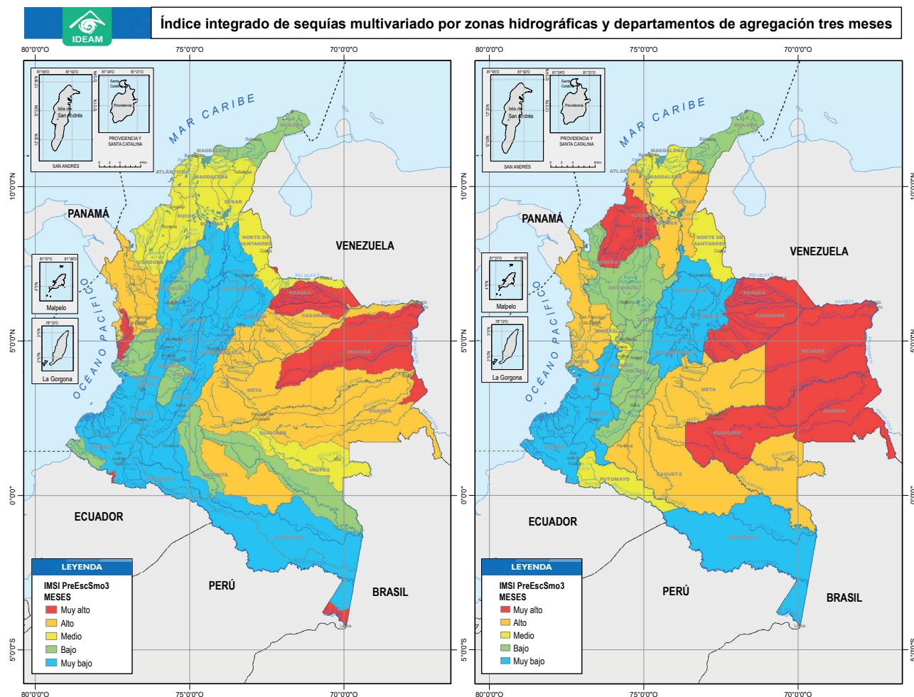
Figura 13. Índice integrado de sequías multivariado por zonas hidrográficas y departamentos agregación tres meses.
