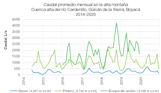
Figura 21. Caudal promedio en los ecosistemas de alta montaña. Casos cuenca Río Claro (izq.), río Cardenillo, Güicán de la Sierra, Boyacá (der.). El caudal de cada ecosistema incluye el (los) del ecosistema inmediatamente superior.
