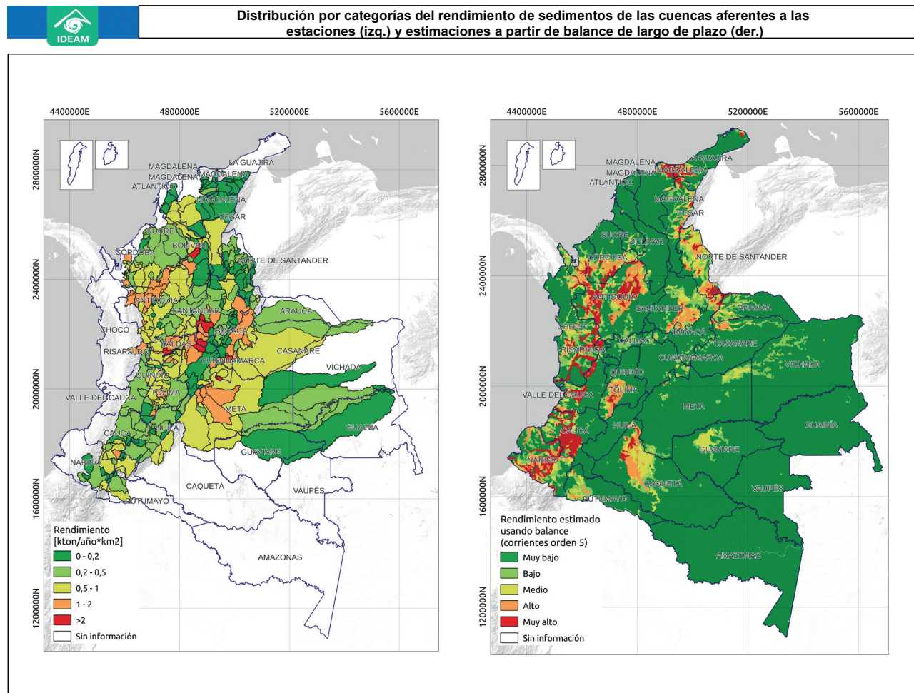
Figura 31. Distribución por categorías del rendimiento de sedimentos de las cuencas aferentes a las estaciones (izq.) y estimaciones a partir de balance de largo plazo (der.).
