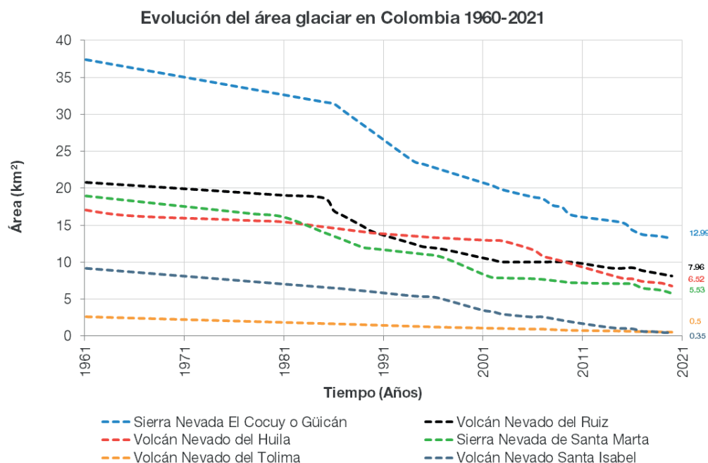
Figura 18. Evolución de la cobertura glaciar en Colombia en las últimas seis décadas.
