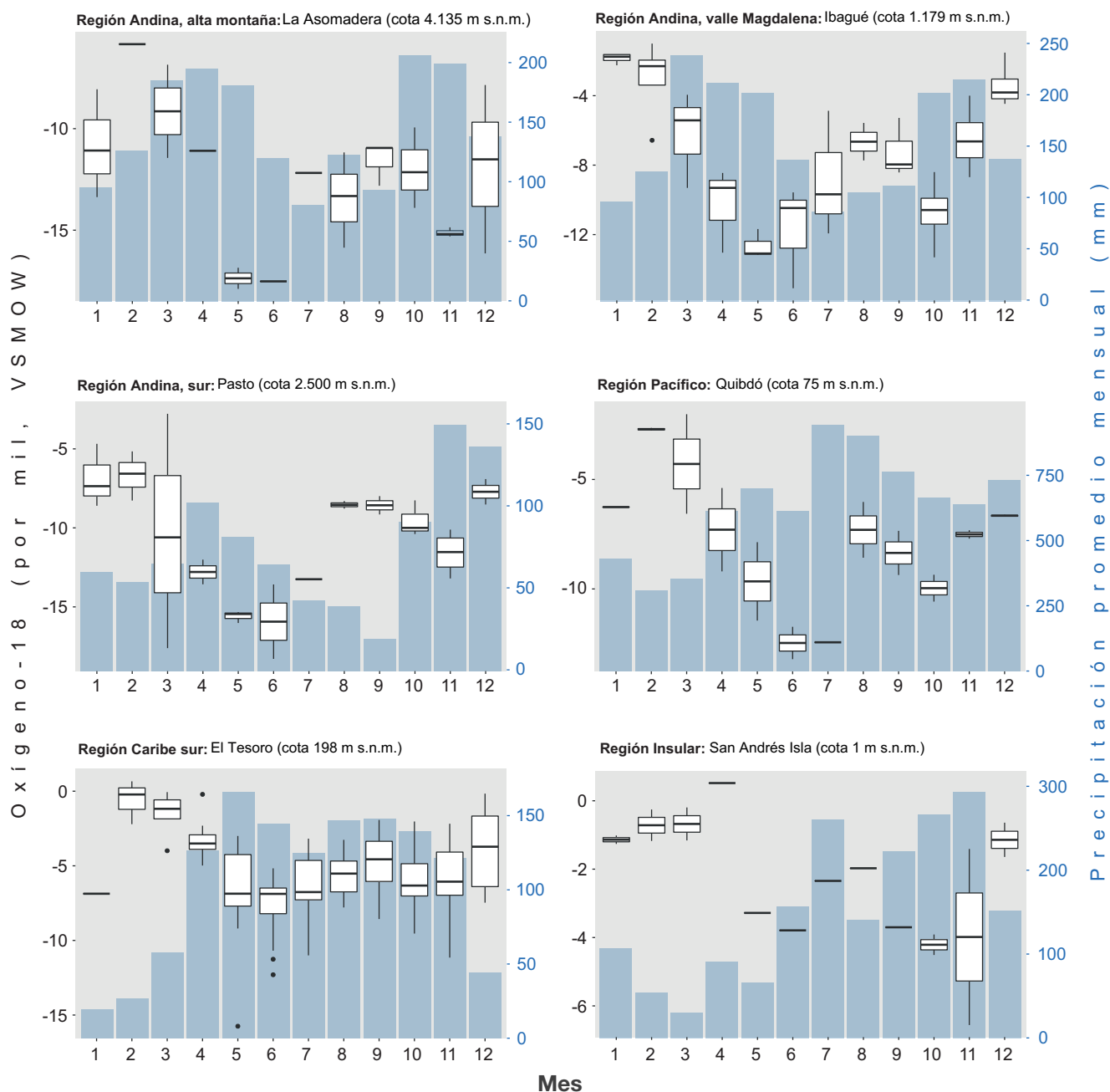
Figura 34. Variación mensual del oxígeno 18 y precipitación, varias estaciones.
