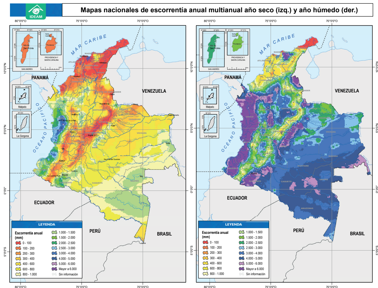
Figura 7. Mapas nacionales de escorrentía anual multianual de año seco (izq.) y año húmedo (der.).
