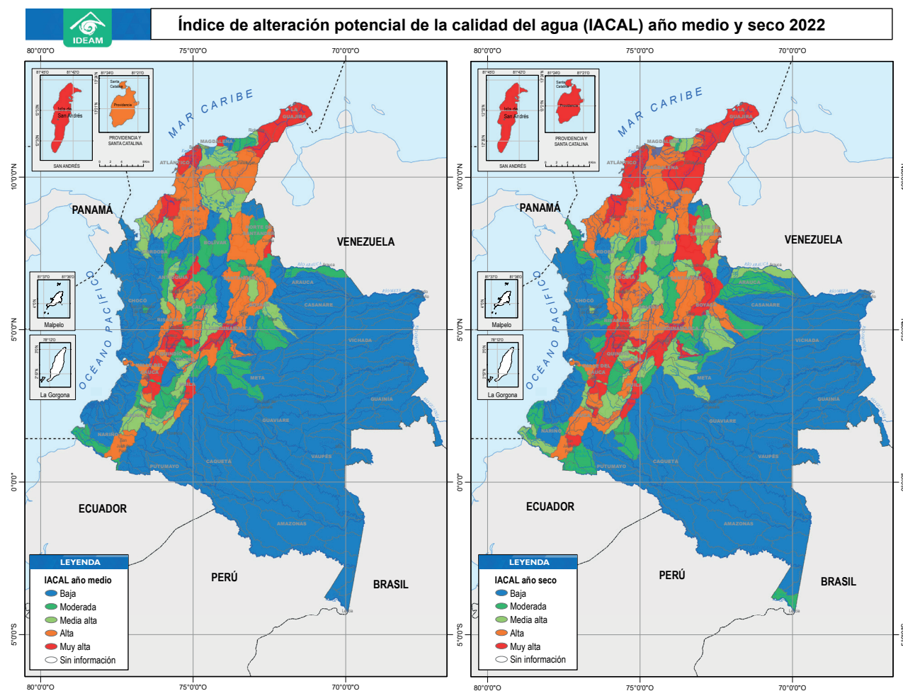
Figura 55. Índice de alteración potencial de la calidad del agua (IACAL) año medio y seco, 2022.
