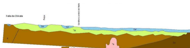
Corte sistema acuífero de Duitama (2)
