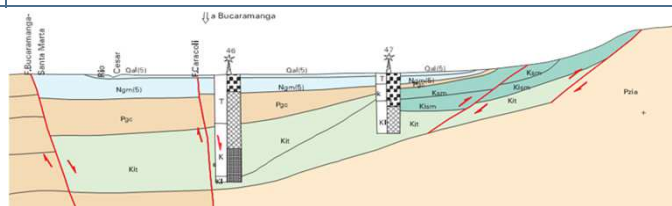
Corte hidrogeológico esquemático (1)
