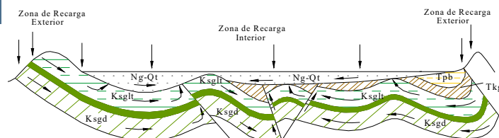
Corte hidrogeológico esquemático de la Sabana de Bogotá (6)
