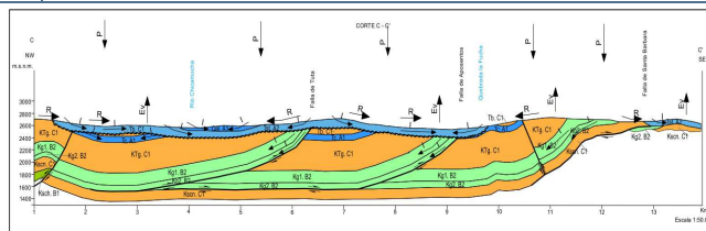
Corte Hidrogeológico Zona Norte - Sector Municipio de Tuta (3)
