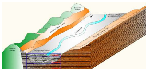
Condición de puntos de agua y Condiciones generales de los PAS-Bloque diagrama del Acuífero del Río Risaralda (1).
