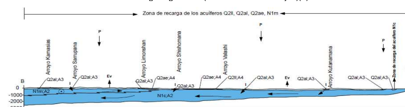
Corte hidrogeológico B-B' (sector NE Media Guajira)(6)
