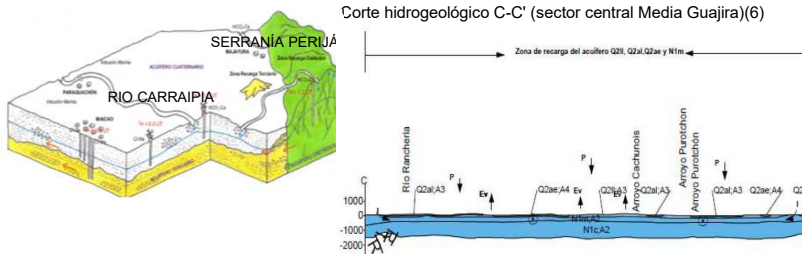
Corte hidrogeológico C-C' (sector central Media Guajira)(6)
