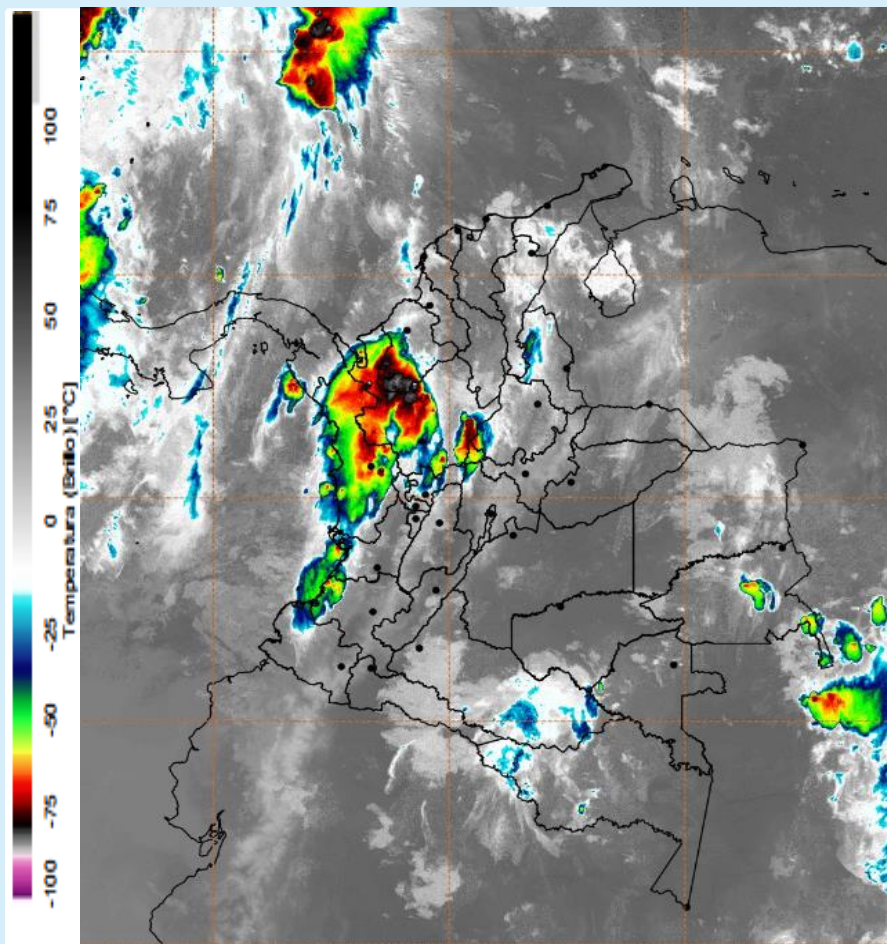
Imagen GOES 16 (East) Canal Infrarrojo | Fuente: RAMMB -GOES 25 de septiembre de 2024 - Hora 23:10 HLC
