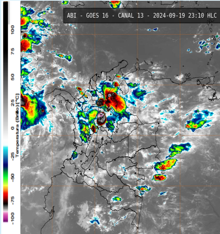
Imagen GOES 16 (East) Canal Infrarrojo | Fuente: IDEAM -GOES 19 de septiembre de 2024 - Hora 23:10 HLC
