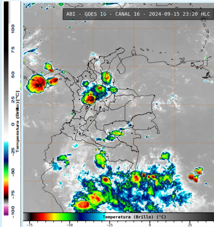
Imagen GOES 16 (East) Canal Infrarrojo | Fuente: IDEAM -GOES 15 de septiembre de 2024 - Hora 23:20 HLC
