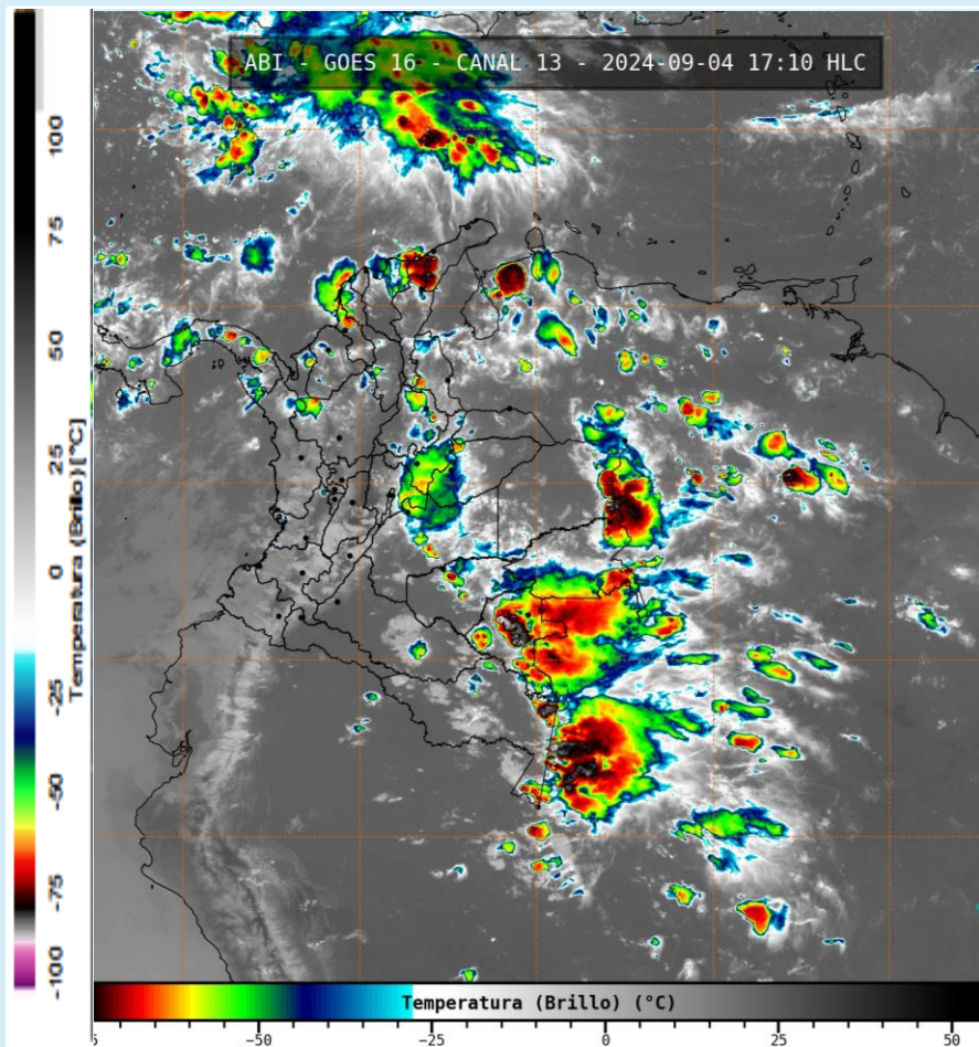
Imagen GOES 16 (East) Canal Infrarrojo | Fuente: IDEAM 4 de septiembre de 2024 - Hora 17:10 HLC
