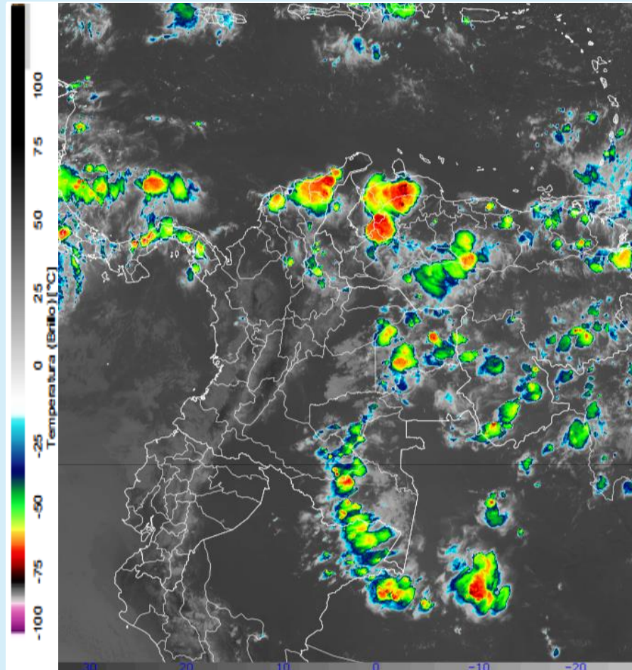
Imagen GOES 16 (East) Canal Infrarrojo | Fuente: GOES-IDEAM 30 de agosto de 2024 - Hora 17:10 HLC
