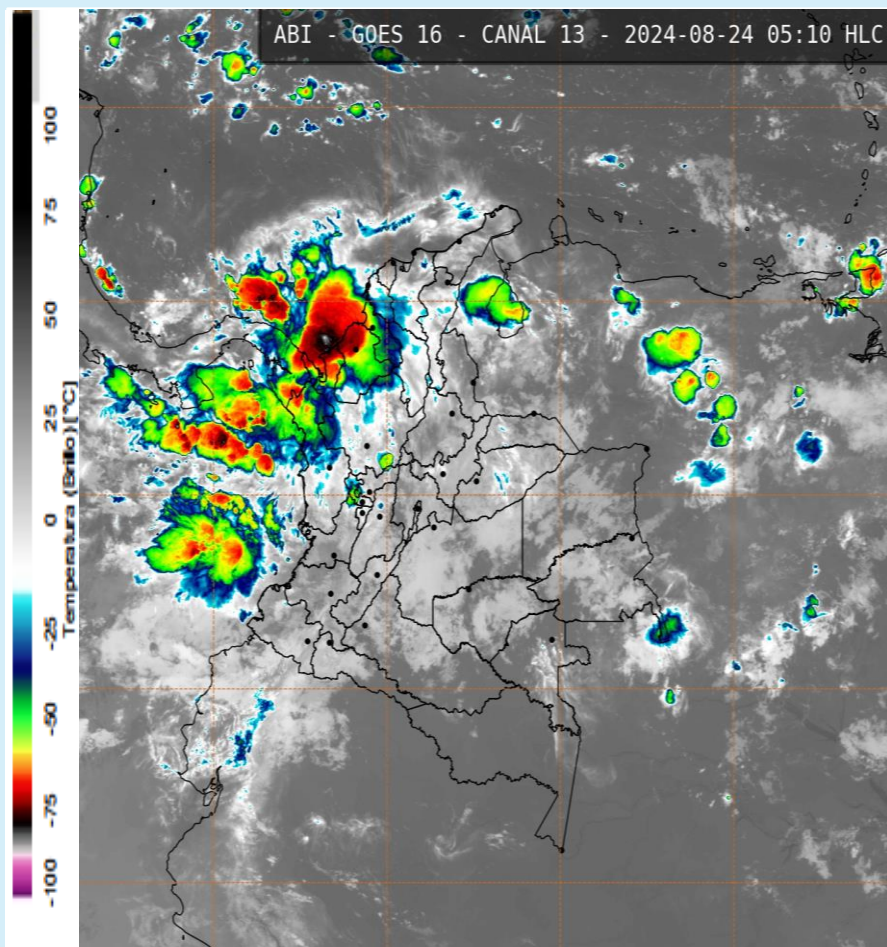
Imagen GOES 16 (East) Canal Infrarrojo | Fuente: GOES-IDEAM 24 de agosto de 2024 - Hora 05:10 HLC
