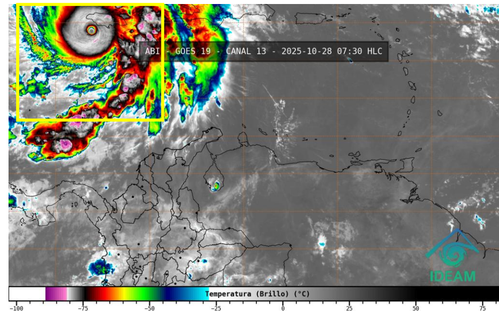
Imagen Satelital GOES -19. Canal Infrarrojo. octubre 28 de 2025, 07:30 HLC Fuente: GOES-IDEAM
