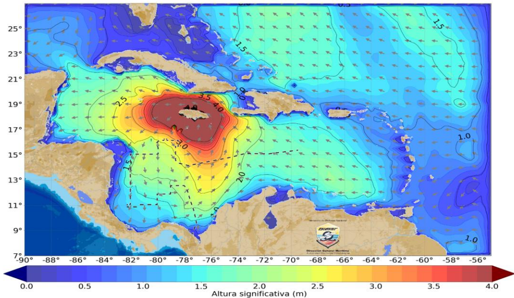
Altura y Dirección de la Ola 28-Oct-2025 12:00hrs (WW3) Cuenca Caribe Colombiana - CCC
