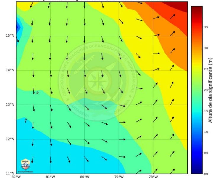
Campo de Altura y Dirección de la Ola 1200R 20251028
