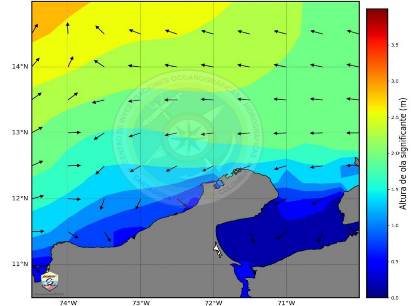
Campo de Altura y Dirección de la Ola 0000R 20251027
