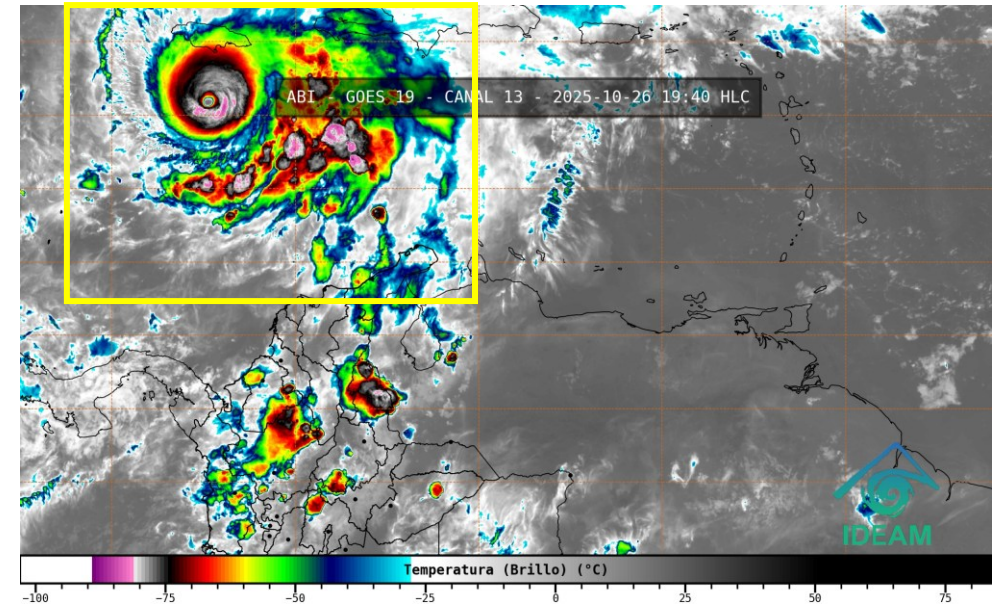
Imagen Satelital GOES -19. Canal Infrarrojo. octubre 26 de 2025, 19:40 HLC Fuente: GOES-IDEAM
