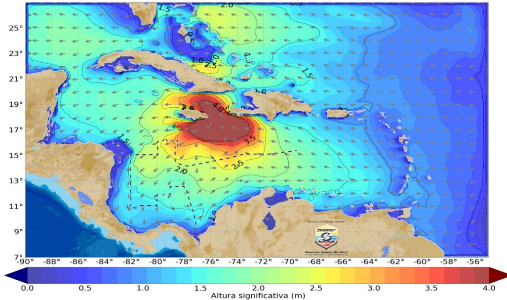
Altura y Dirección de la Ola 27-Oct-2025 00:00hrs (WW3) Cuenca Caribe Colombiana - CCC
