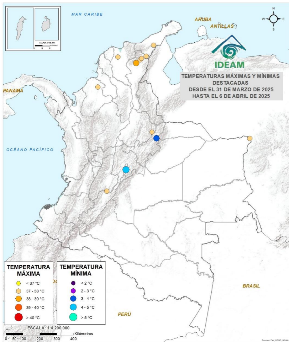
Temperaturas mínima y máxima del aire destacadas del 31 de marzo al 6 de abril de 2025
