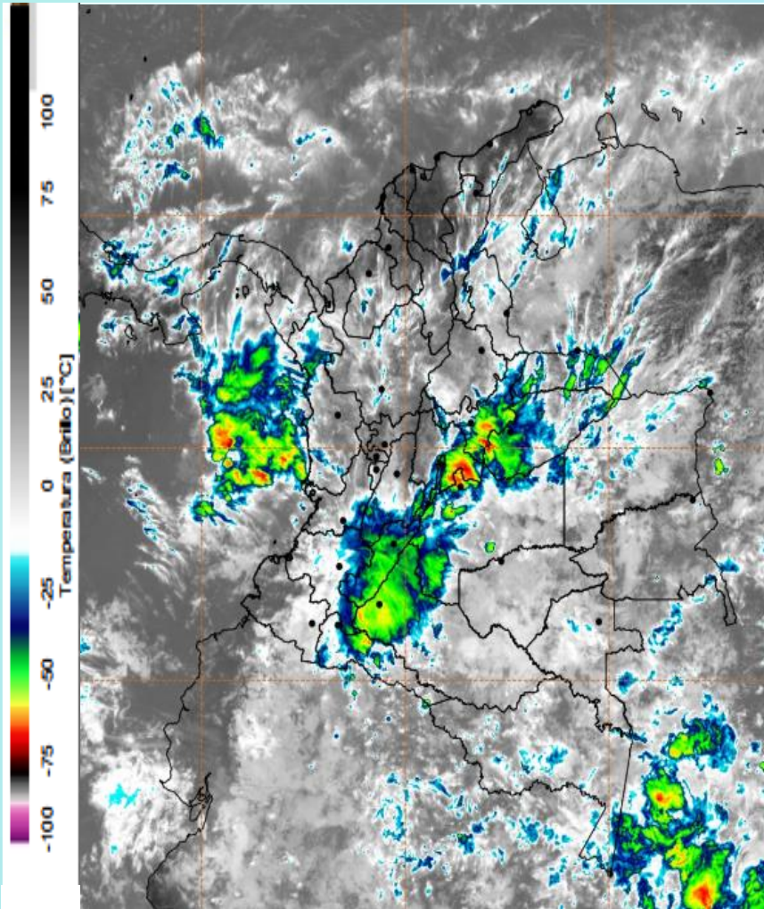
Imagen GOES East Canal Infrarrojo, 2 de abril de 2025 - Hora 16:50 HLC. Fuente: RAMMB-SLIDER
