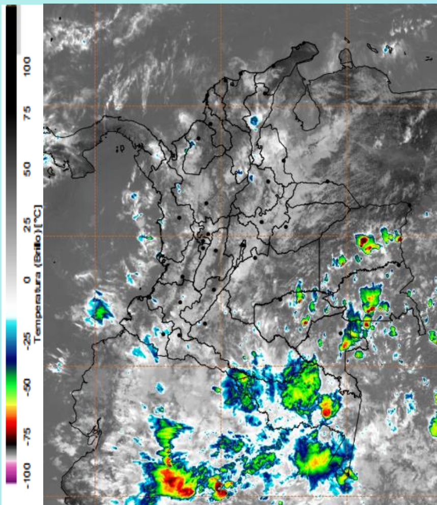
Imagen GOES East Canal Infrarrojo, 1 de abril de 2025 - Hora 12:00 HLC. Fuente: RAMMB-SLIDER
