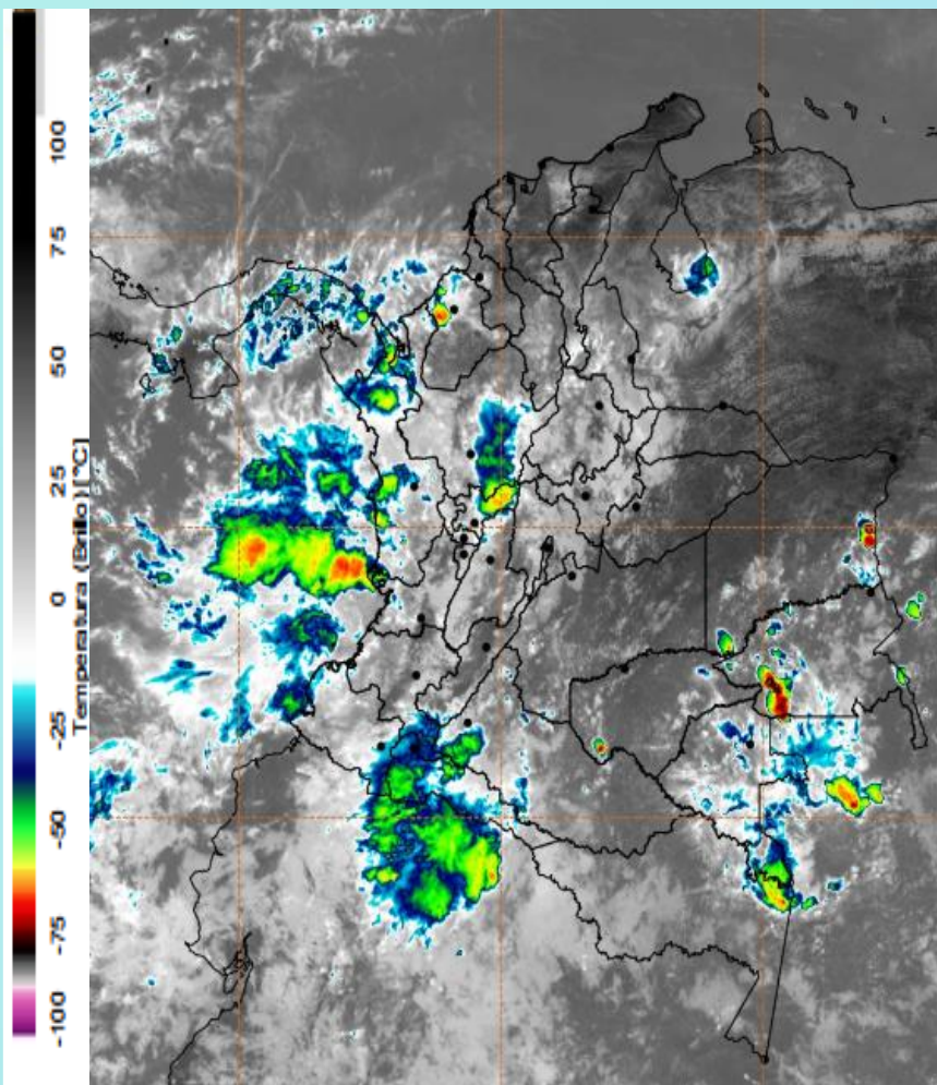
Imagen GOES East Canal Infrarrojo, 28 de marzo de 2025 - Hora 12:00 HLC. Fuente: GOES 16
