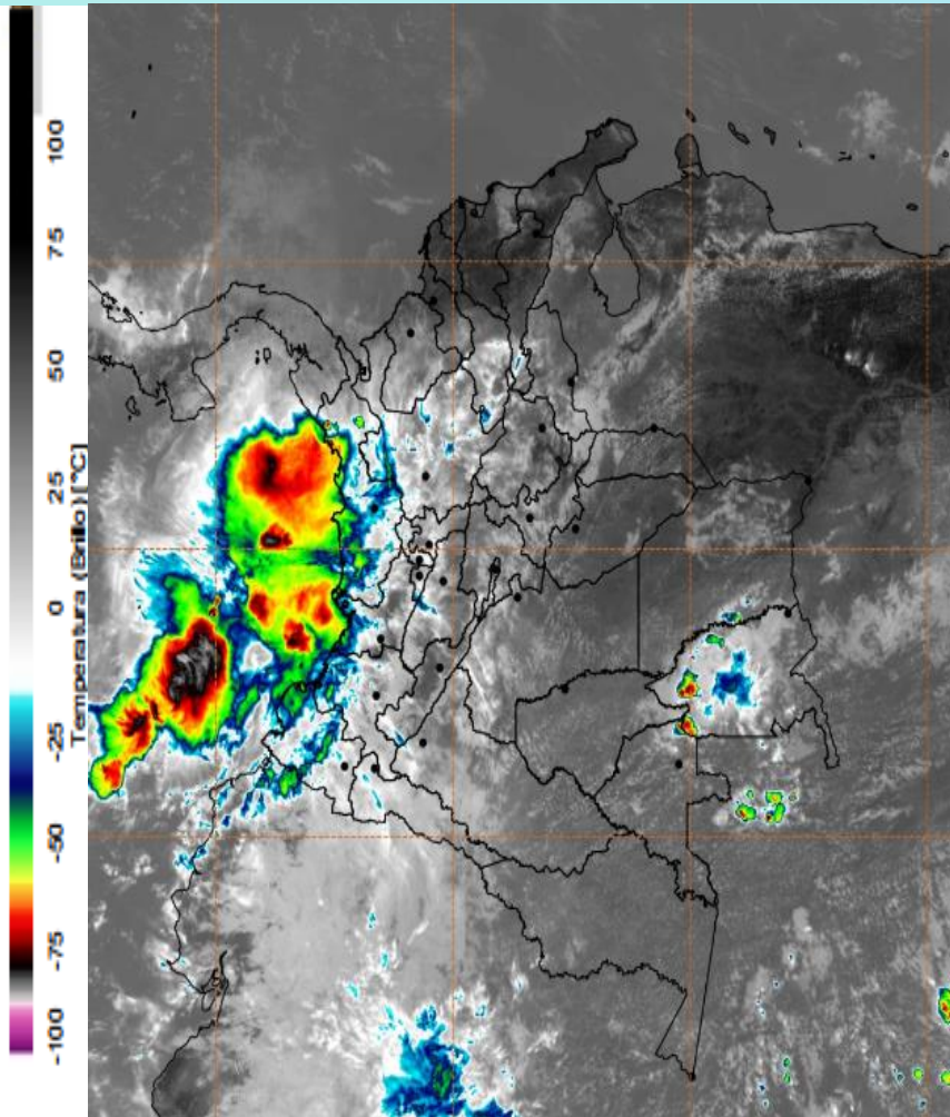
Imagen GOES East Canal Infrarrojo, 23 de marzo de 2025 - Hora 11:40 HLC. Fuente: GOES 16
