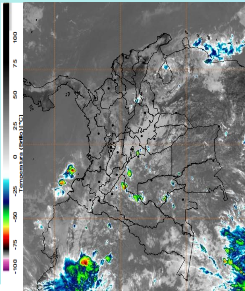
Imagen GOES East Canal Infrarrojo, 19 de marzo de 2025 - Hora 11:50 HLC. Fuente: GOES 16
