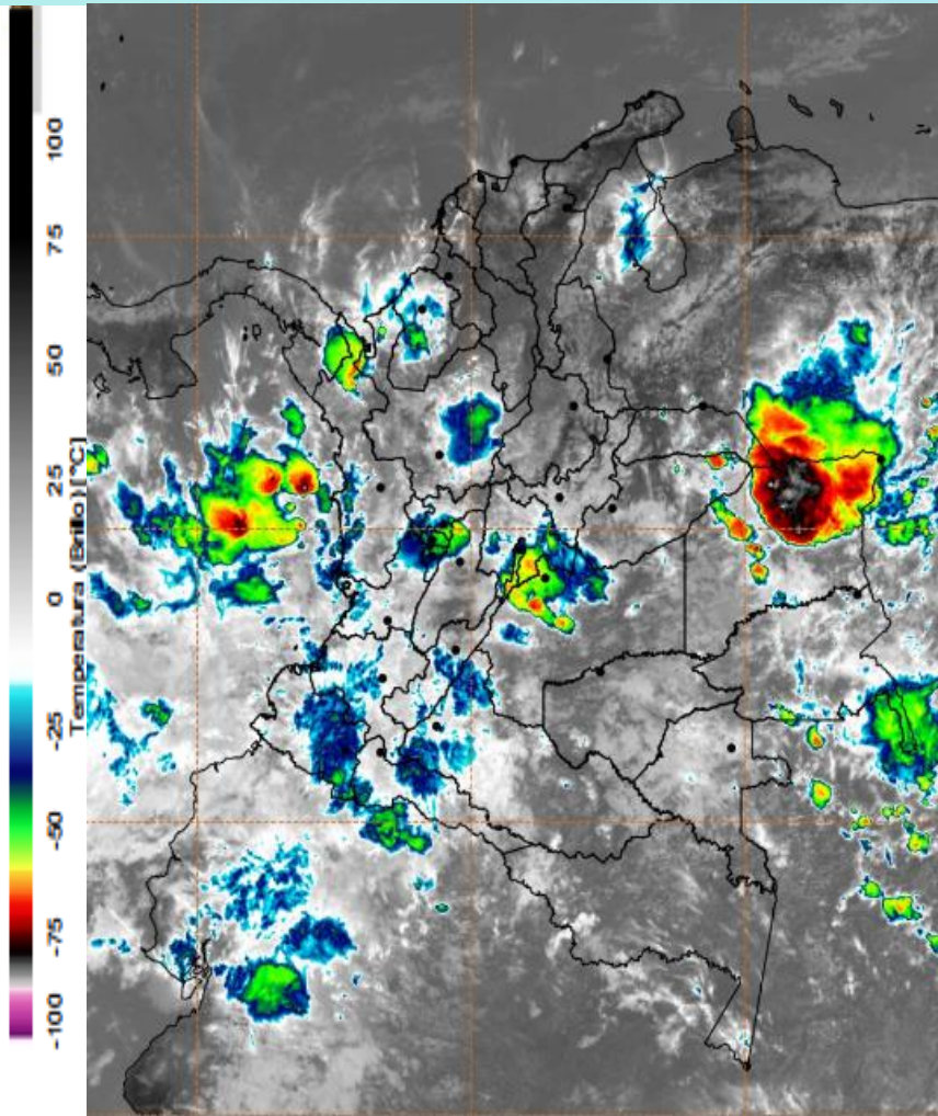
Imagen GOES East Canal Infrarrojo, 17 de marzo de 2025 - Hora 11:50 HLC. Fuente: GOES 16
