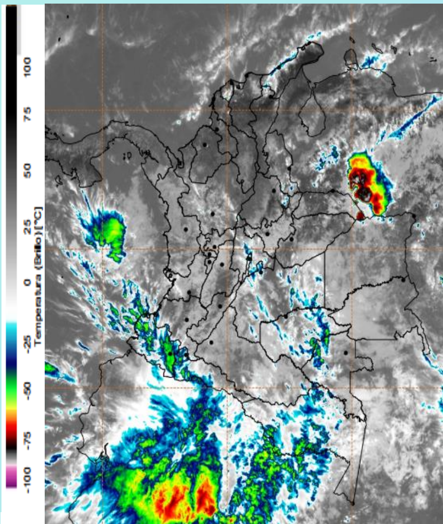
Imagen GOES East Canal Infrarrojo, 15 de marzo de 2025 - Hora 11:50 HLC. Fuente: GOES 16
