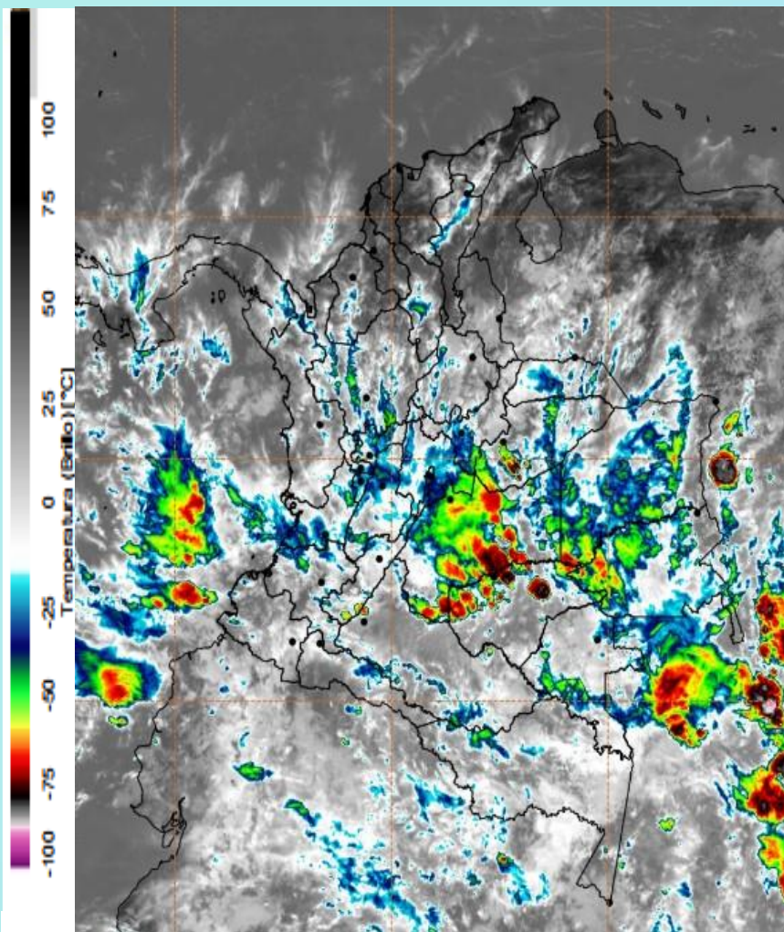
Imagen GOES East Canal Infrarrojo, 14 de marzo de 2025 - Hora 11:50 HLC. Fuente: GOES 16
