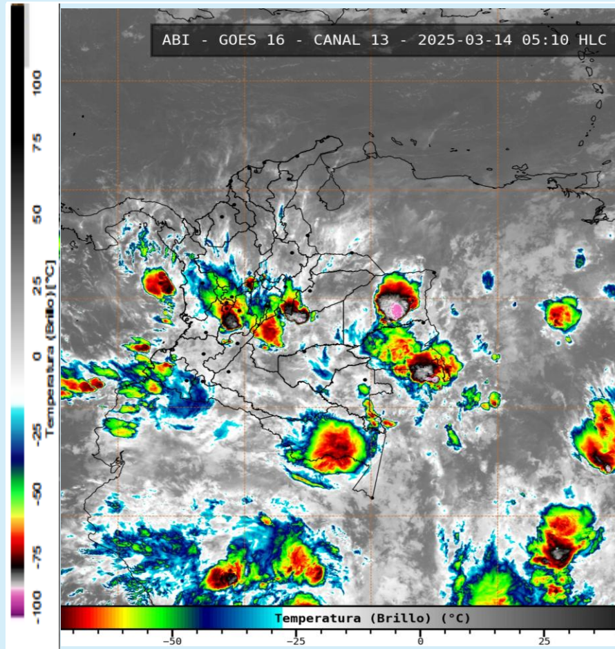
Imagen GOES 16 (East) Canal Infrarrojo 14 de marzo de 2025 - Hora 05:10 HLC Fuente: IDEAM
