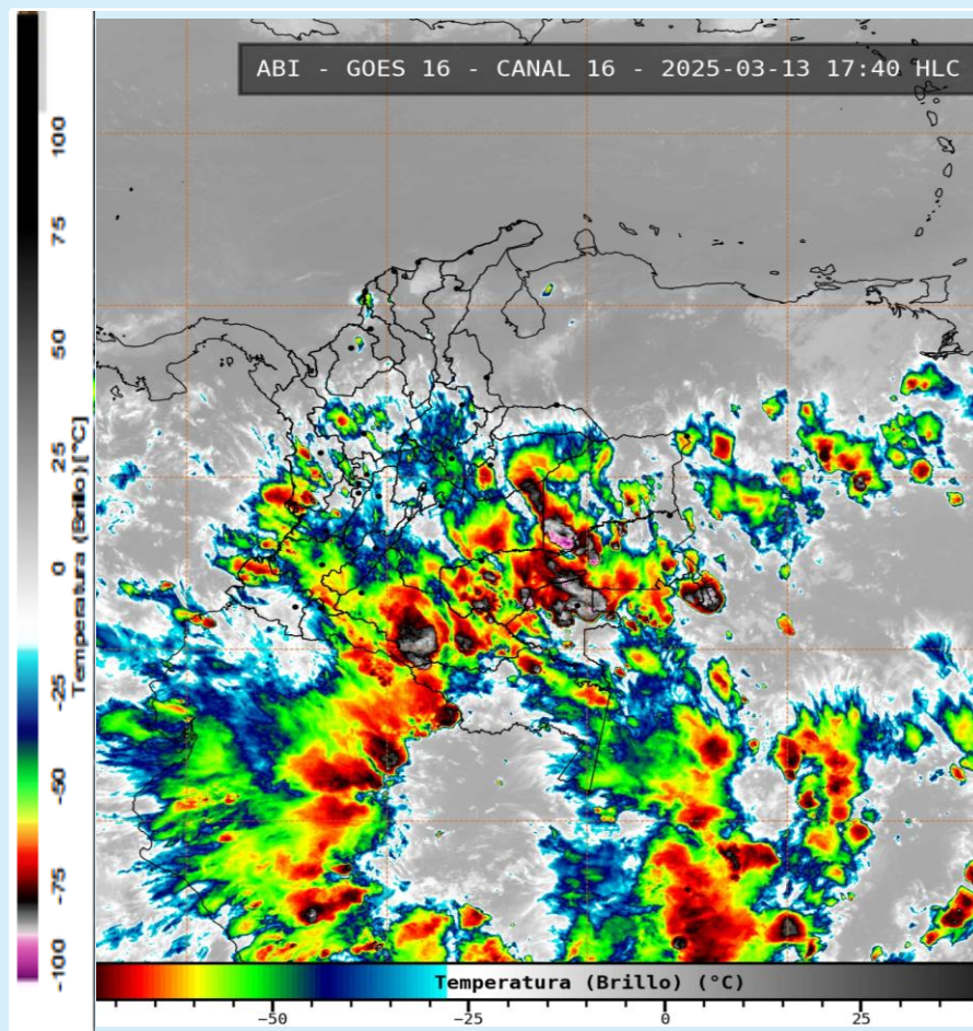
Imagen GOES 16 (East) Canal Infrarrojo 13 de marzo de 2025 - Hora 17:40 HLC Fuente: IDEAM
