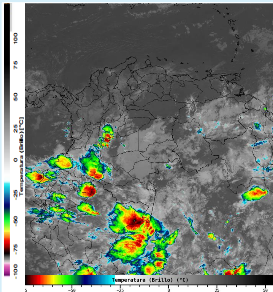
Imagen GOES 16 (East) Canal Infrarrojo 13 de marzo de 2025 - Hora 05:10 HLC Fuente: IDEAM
