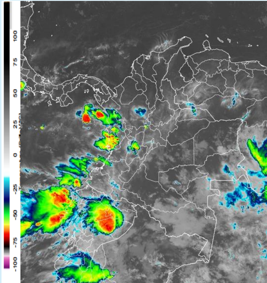
Imagen GOES 16 (East) Canal Infrarrojo 11 de marzo de 2025 - Hora 17:10 HLC
