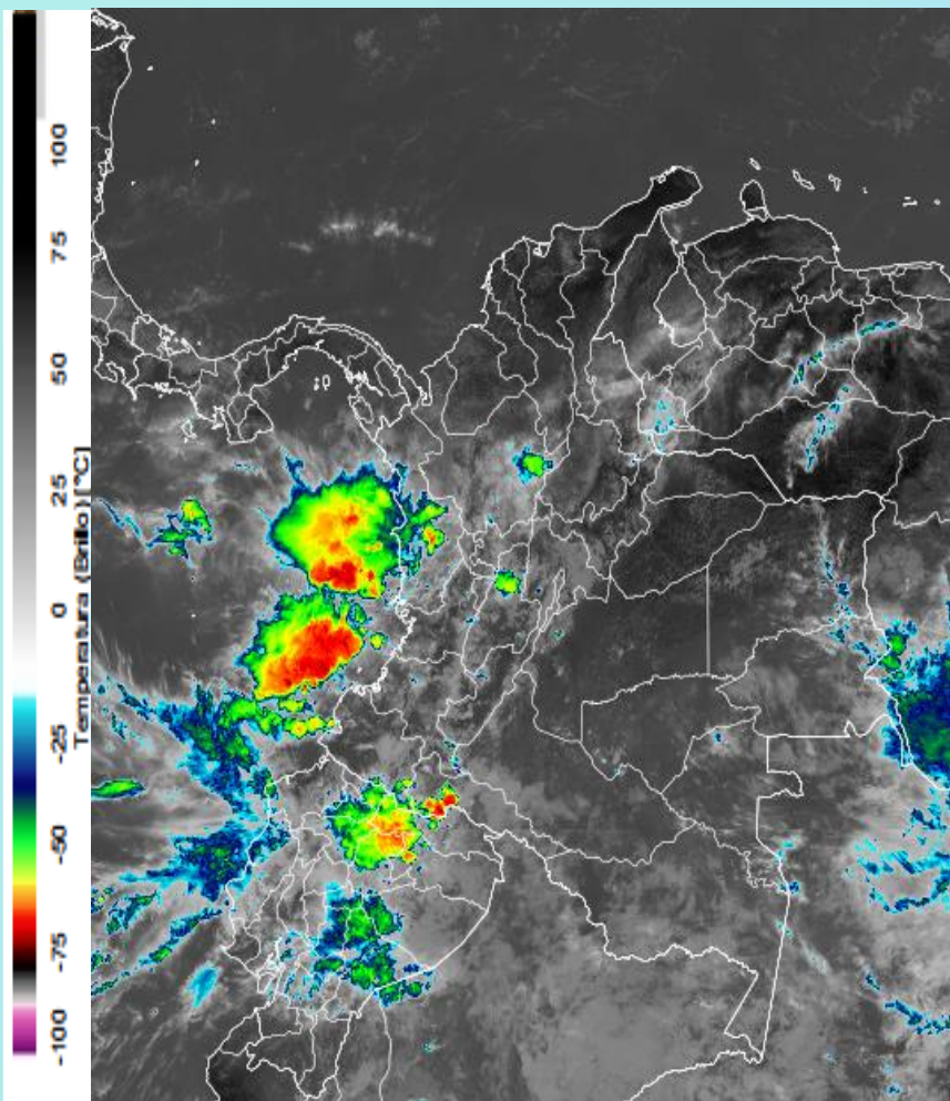
Imagen GOES East Canal Infrarrojo, 11 de marzo de 2025 - Hora 11:20 HLC. Fuente: GOES 16
