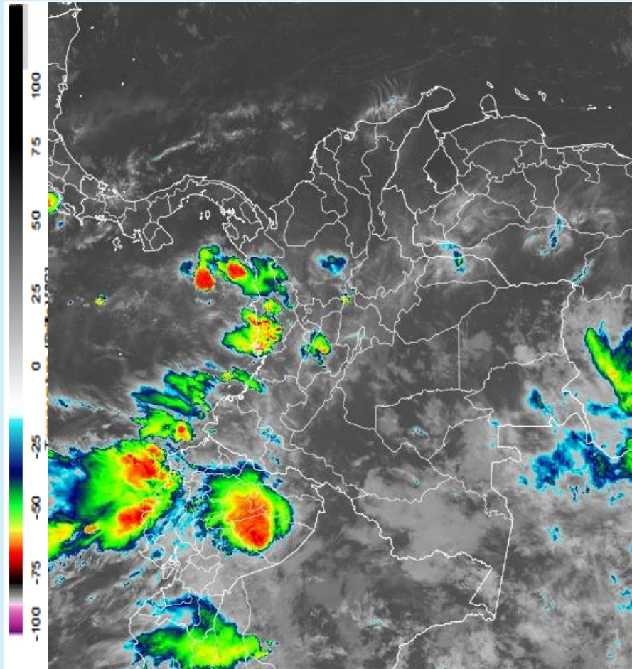
Imagen GOES 16 (East) Canal Infrarrojo 11 de marzo de 2025 - Hora 05:10 HLC
