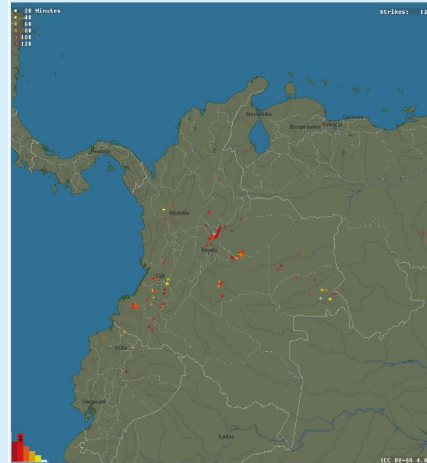
Descargas eléctricas en las últimas 4 horas Fuente: https://www.blitzortung.org/
