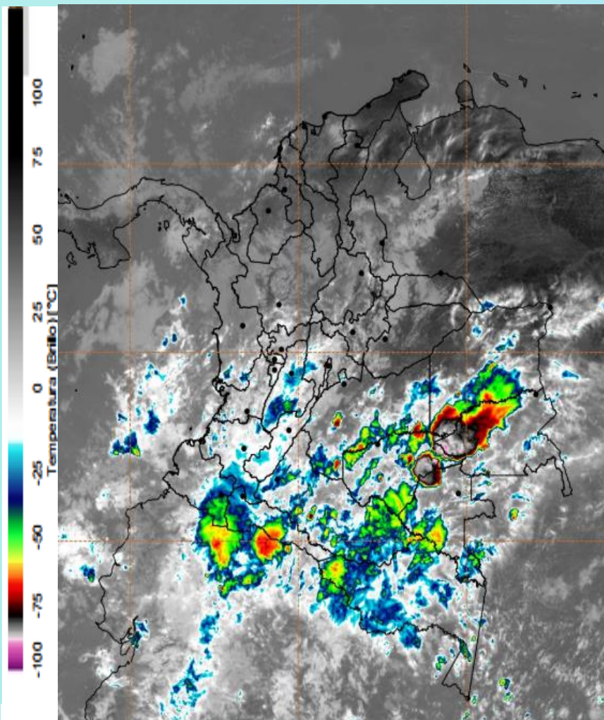
Imagen GOES East Canal Infrarrojo, 27 de febrero de 2025 - Hora 11:50 HLC. Fuente: GOES 16
