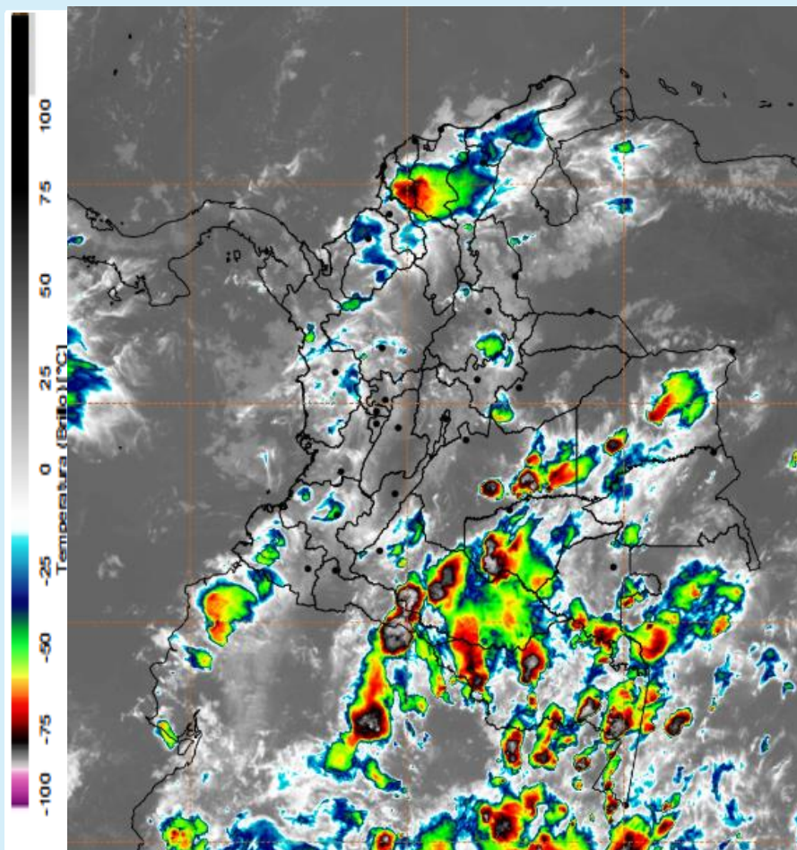
Imagen GOES 16 (East) Canal Infrarrojo 26 de Febrero de 2025- Hora 18:00 HLC Fuente: IDEAM
