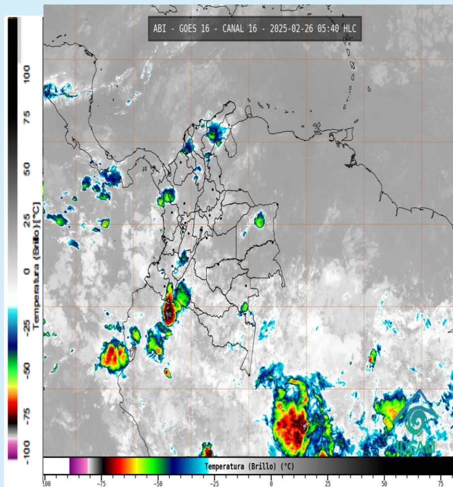
Imagen GOES 16 (East) Canal Infrarrojo 26 de Febrero de 2025- Hora 05:40 HLC Fuente: IDEAM
