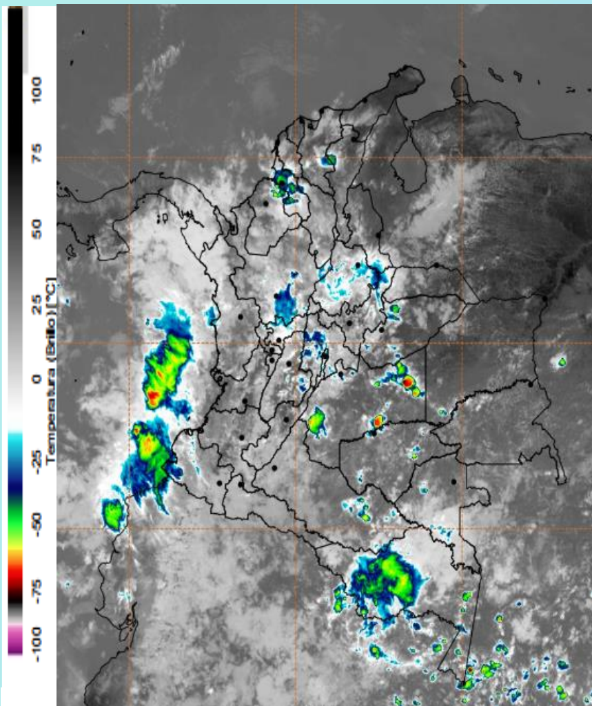
Imagen GOES East Canal Infrarrojo, 25 de febrero de 2025 - Hora 11:50 HLC. Fuente: GOES 16
