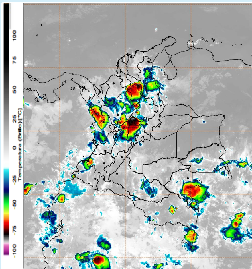
Imagen GOES 16 (East) Canal Infrarrojo 24 de febrero de 2025 - Hora 23:20 HLC Fuente: IDEAM
