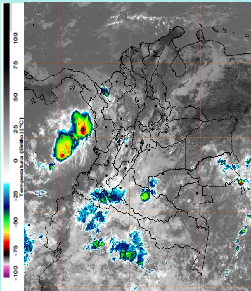
Imagen GOES East Canal Infrarrojo, 24 de febrero de 2025 - Hora 11:40 HLC. Fuente: GOES 16
