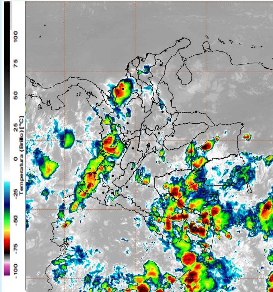
Imagen GOES 16 (East) Canal Infrarrojo 23 de febrero de 2025 - Hora 17:40 HLC Fuente: IDEAM
