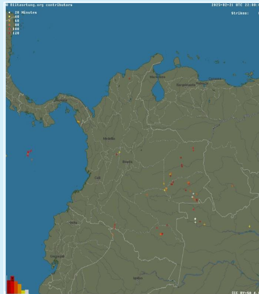
Descargas eléctricas en las últimas 3 horas Fuente: https://map.blitzortung.org/#google_vignette
