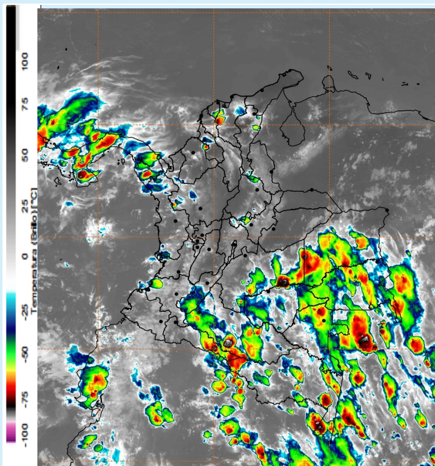
Imagen GOES 16 (East) Canal Infrarrojo 20 de febrero de 2025 - Hora 17:30 HLC Fuente: IDEAM
