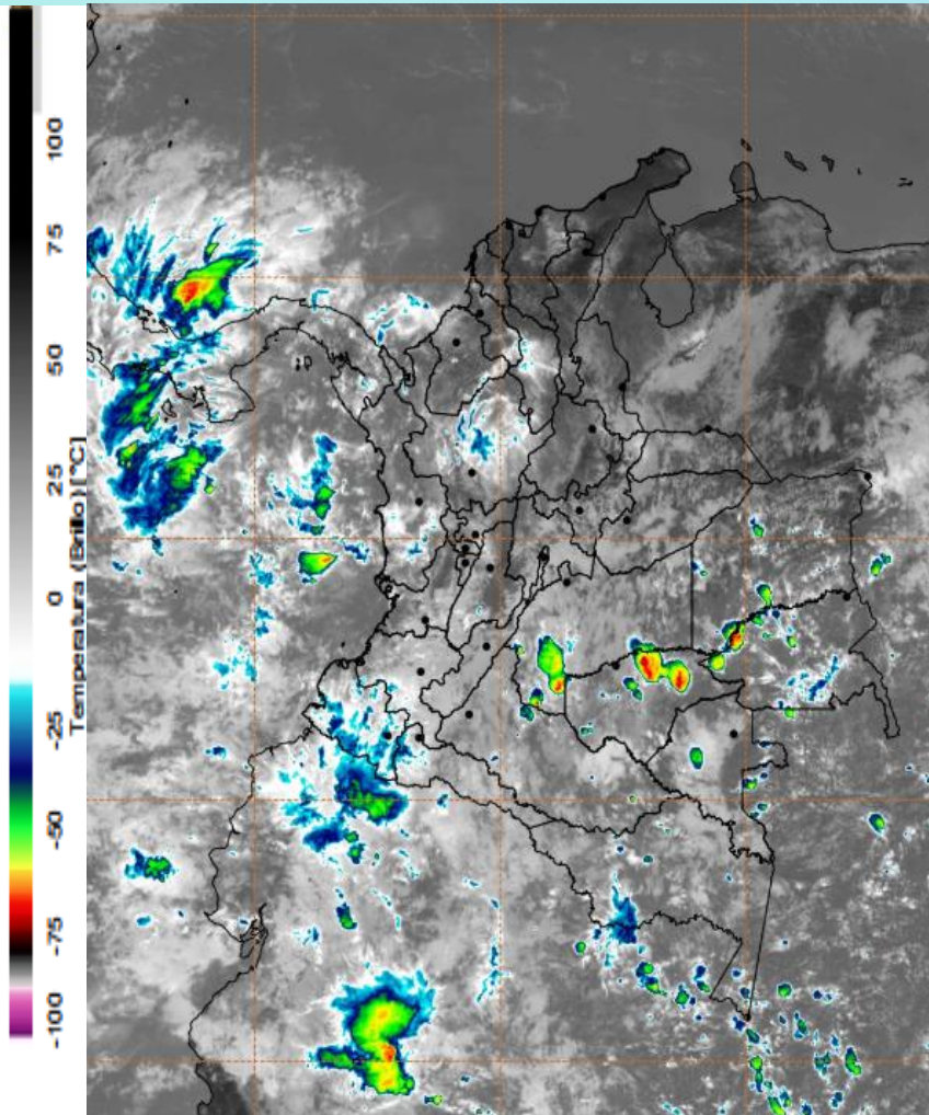
Imagen GOES East Canal Infrarrojo, 20 de febrero de 2025 - Hora 11:50 HLC. Fuente: GOES 16
