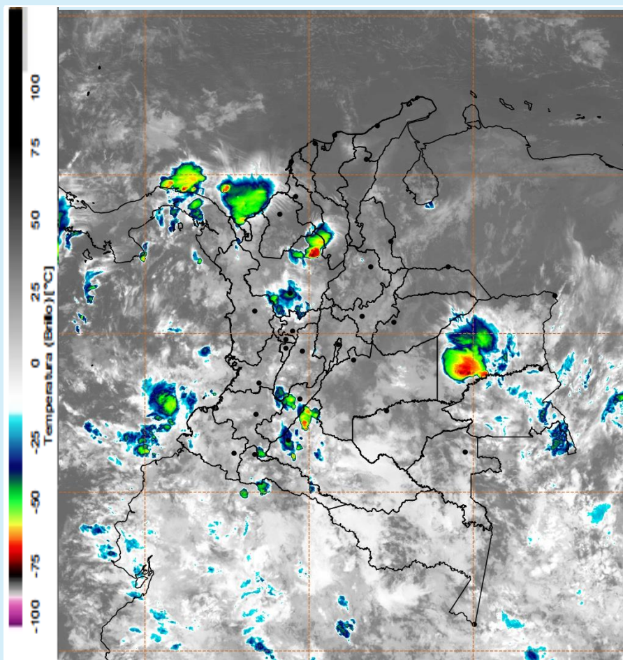
Imagen GOES 16 (East) Canal Infrarrojo 19 de febrero de 2025 - Hora 04:40 HLC Fuente: IDEAM
