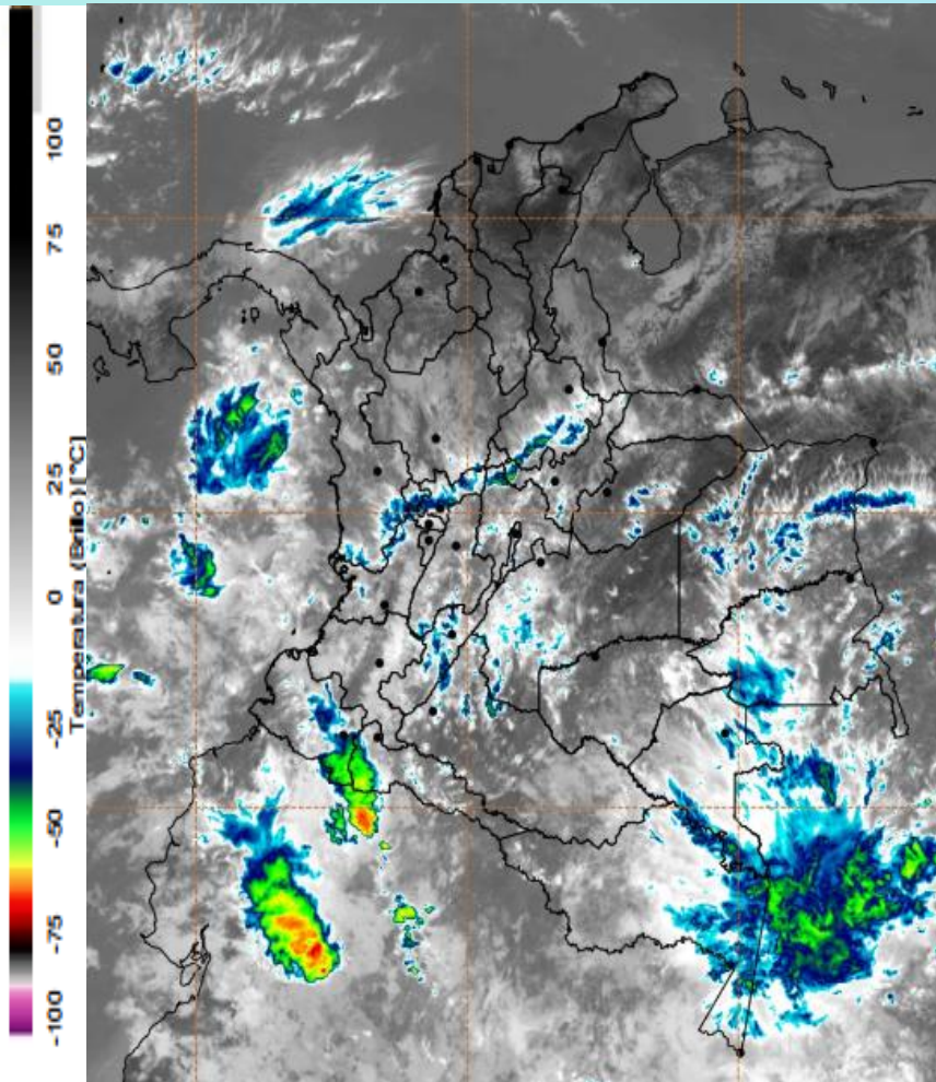
Imagen GOES East Canal Infrarrojo, 18 de febrero de 2025 - Hora 11:50 HLC. Fuente: GOES 16
