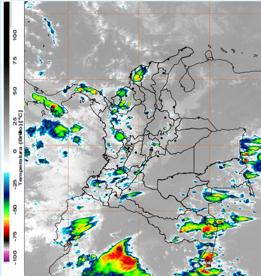
Imagen GOES 16 (East) Canal Infrarrojo 16 de febrero de 2025 - Hora 17:30 HLC Fuente: IDEAM
