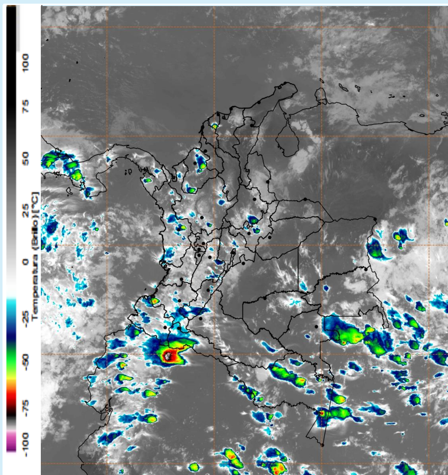
Imagen GOES 16 (East) Canal Infrarrojo 15 de febrero de 2025 - Hora 17:10 HLC Fuente: IDEAM
