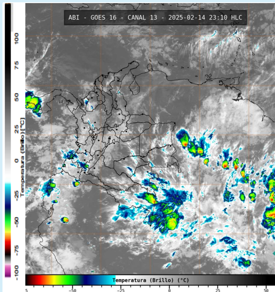
Imagen GOES 16 (East) Canal Infrarrojo 14 de febrero de 2025 - Hora 23:10 HLC Fuente: IDEAM
