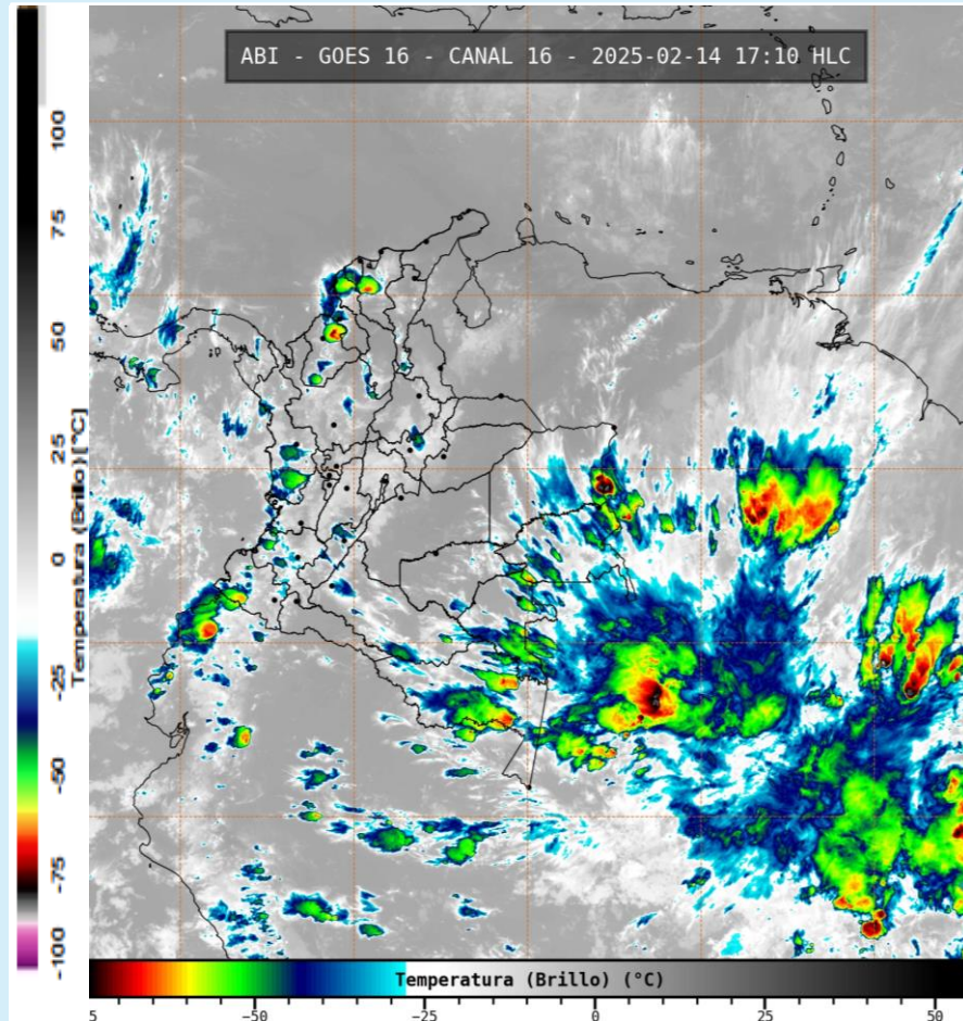
Imagen GOES 16 (East) Canal Infrarrojo 14 de febrero de 2025 - Hora 17:10 HLC Fuente: IDEAM
