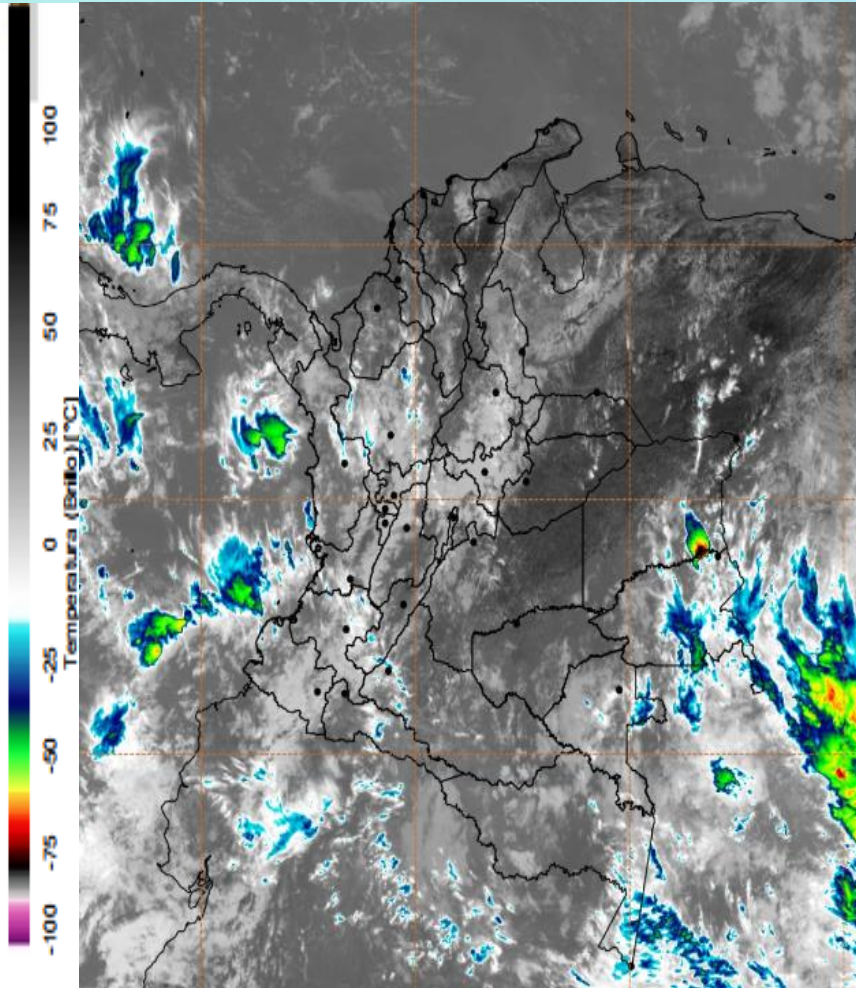
Imagen GOES East Canal Infrarrojo, 14 de febrero de 2025 - Hora 11:50 HLC. Fuente: GOES 16
