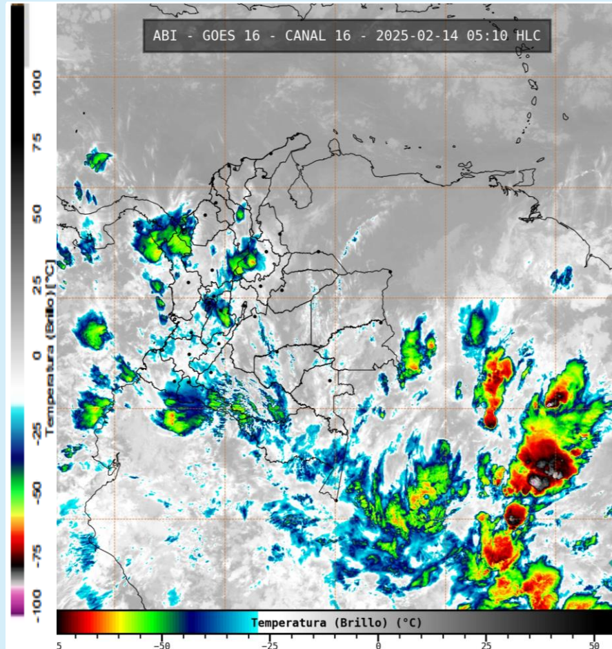
Imagen GOES 16 (East) Canal Infrarrojo 14 de febrero de 2025 - Hora 05:10 HLC Fuente: IDEAM
