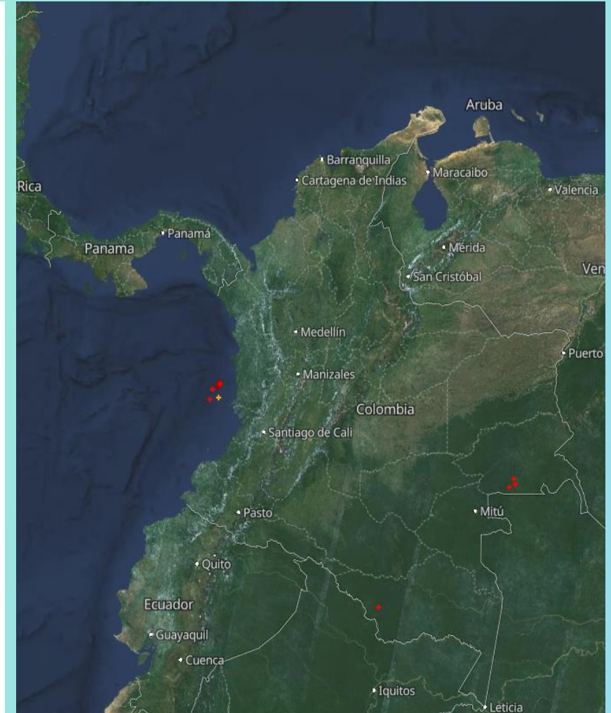
Descargas eléctricas en las últimas dos horas. Fuente: Blitzortung.org - Live Lightning Map
