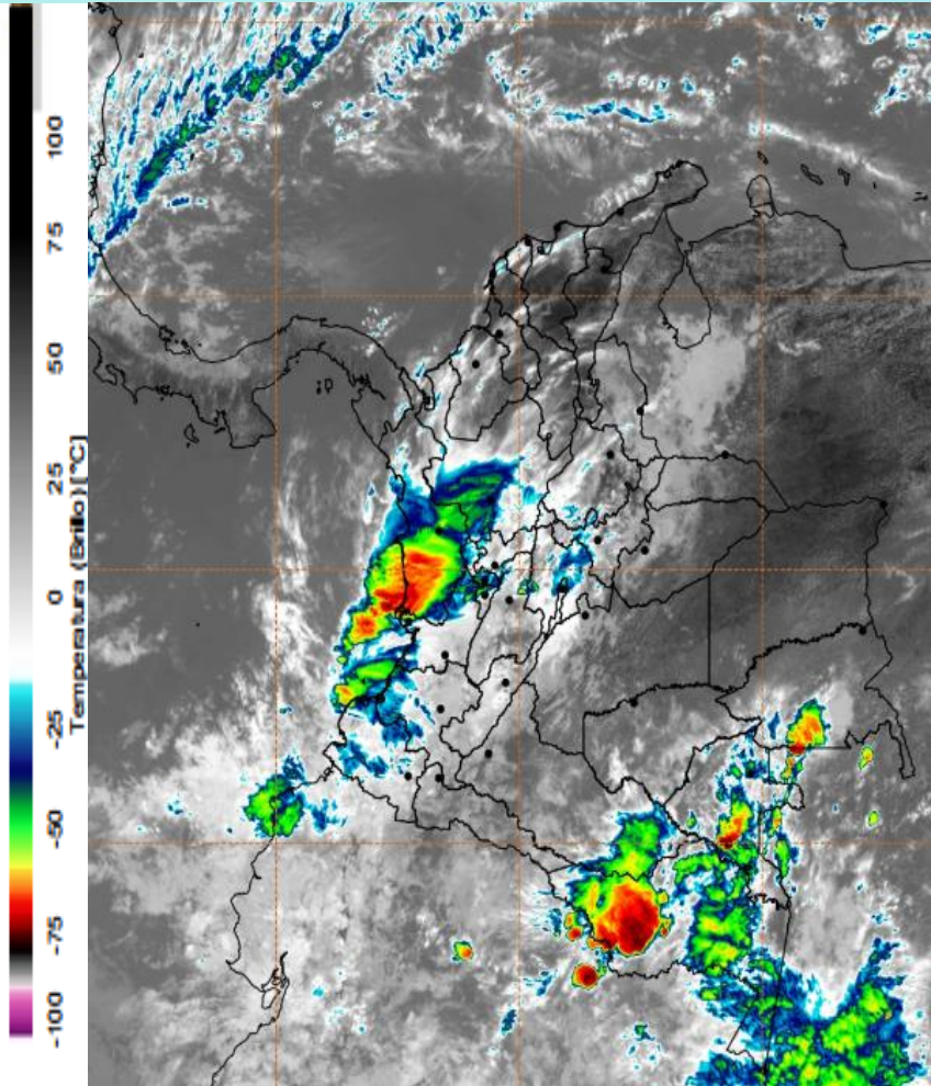
Imagen GOES East Canal Infrarrojo, 11 de febrero de 2025 - Hora 11:40 HLC. Fuente: GOES 16
