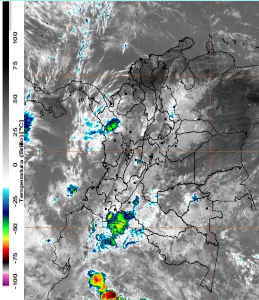
Imagen GOES East Canal Infrarrojo, 10 de febrero de 2025 - Hora 11:40 HLC. Fuente: GOES 16
