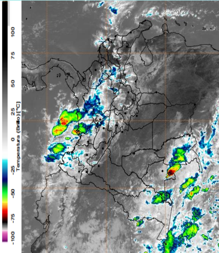
Imagen GOES East Canal Infrarrojo, 5 de febrero de 2025 - Hora 11:20 HLC. Fuente: GOES 16
