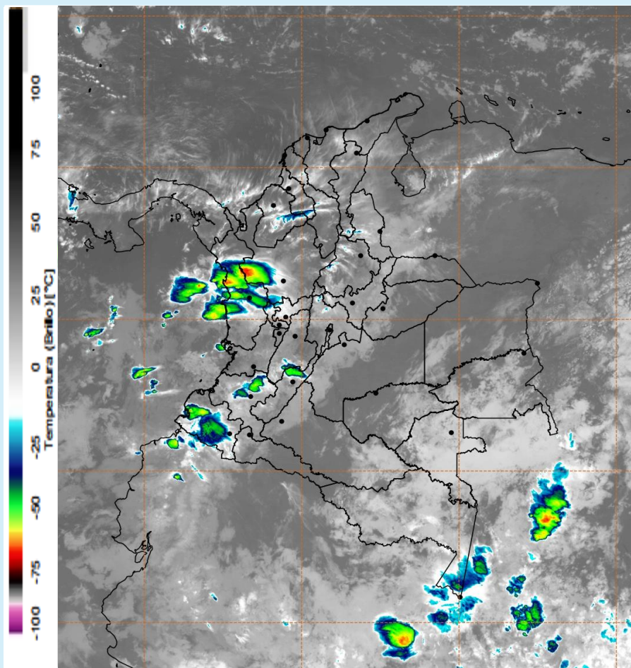
Imagen GOES 16 (East) Canal Infrarrojo 3 de febrero de 2025 - Hora 05:20 HLC Fuente: IDEAM
