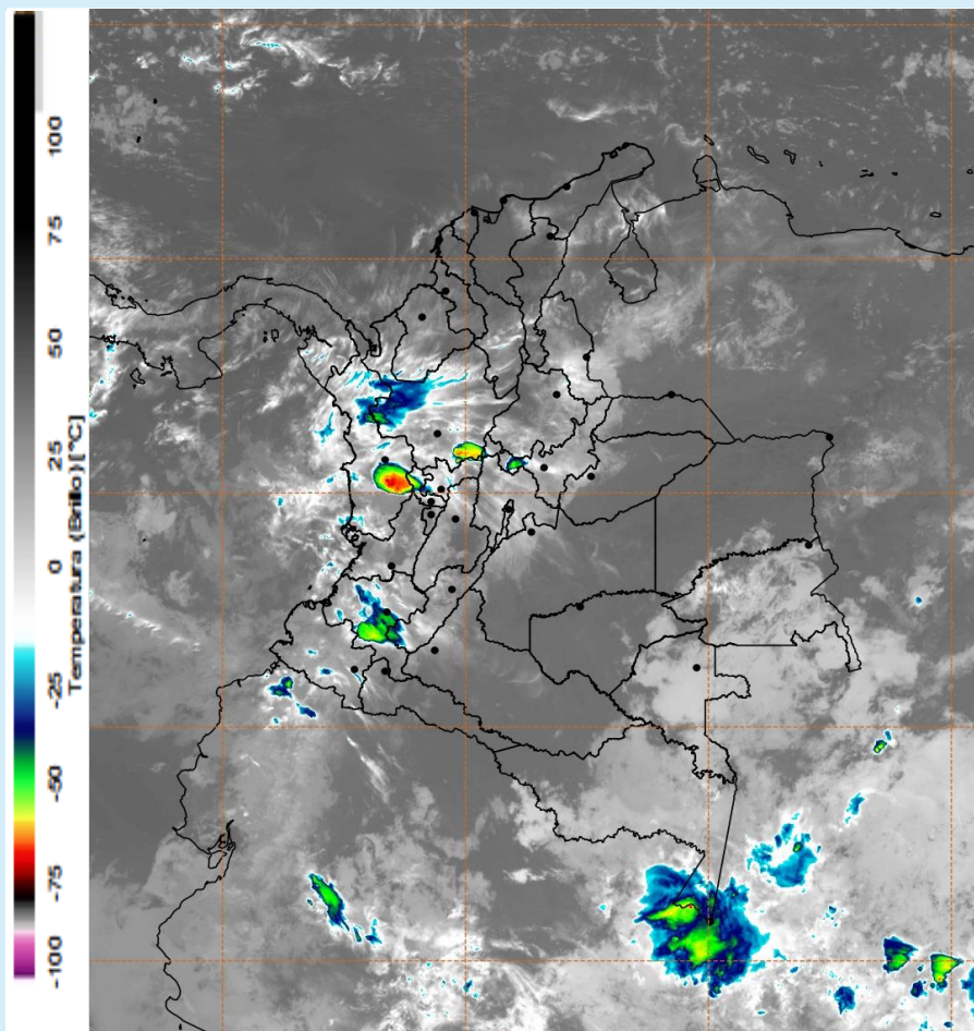
Imagen GOES 16 (East) Canal Infrarrojo 2 de febrero de 2025 - Hora 23:20 HLC Fuente: IDEAM
