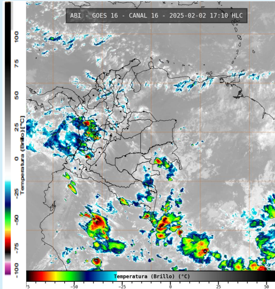
Imagen GOES 16 (East) Canal Infrarrojo 2 de febrero de 2025 - Hora 17:10 HLC Fuente: IDEAM
